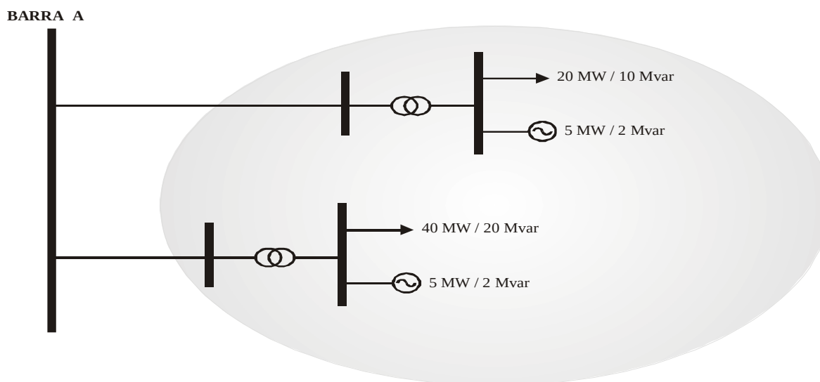
Figura 4 Sistema de potência a ser equivalentado - Geração
